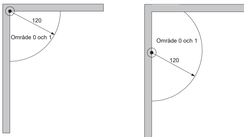
3) Vy från ovan (för olika placering av vattenblandare)
