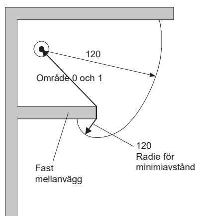
4) Vy från ovan med vattenblandare (med fast mellanvägg och radie för minimiavstånd runt mellanväggen)
