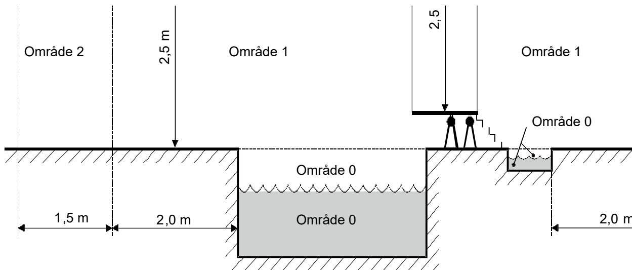
Figur 702A.1 – Områdesindelning för simbassänger och plaskdammar
