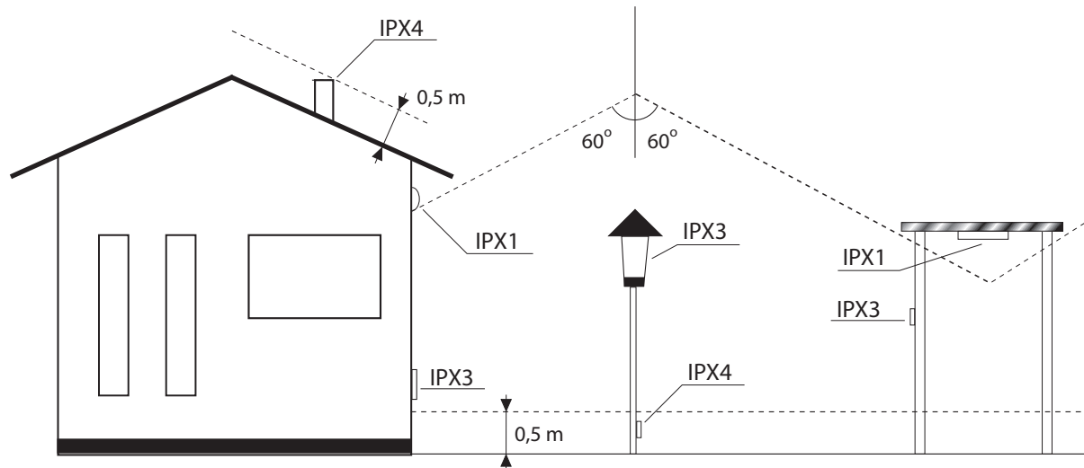
Figur 51.NB.1 – Exempel på kapslingsklasser utomhus
