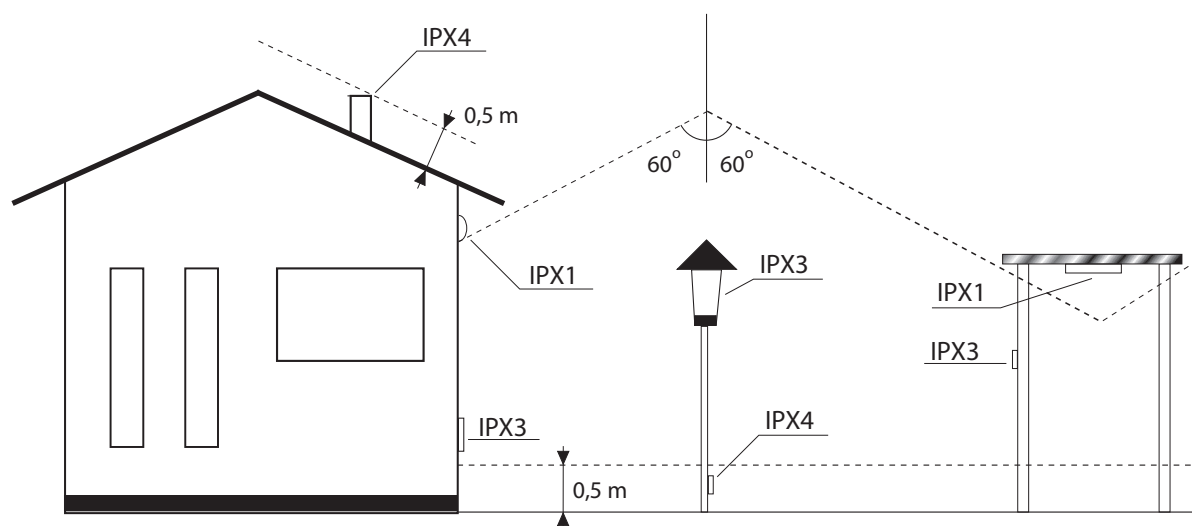
Figur 751A – Exempel på kapslingsklasser utomhus
